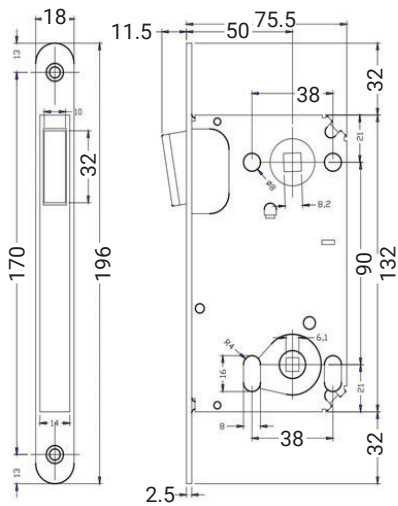
► Cerradura con condena 90 mm
