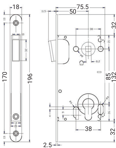
► Cerradura c/bocallave yale 85 mm
